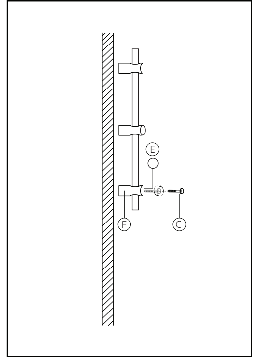
3. เปิดฝาคกรอบเป็นด้านล่าง ( E ) เพื่อนำสกรู ( C ) ใส่ไปด้านในเป็นล่าง ( F ) และขันสกรูยึดแป้นเข้าผนัง
