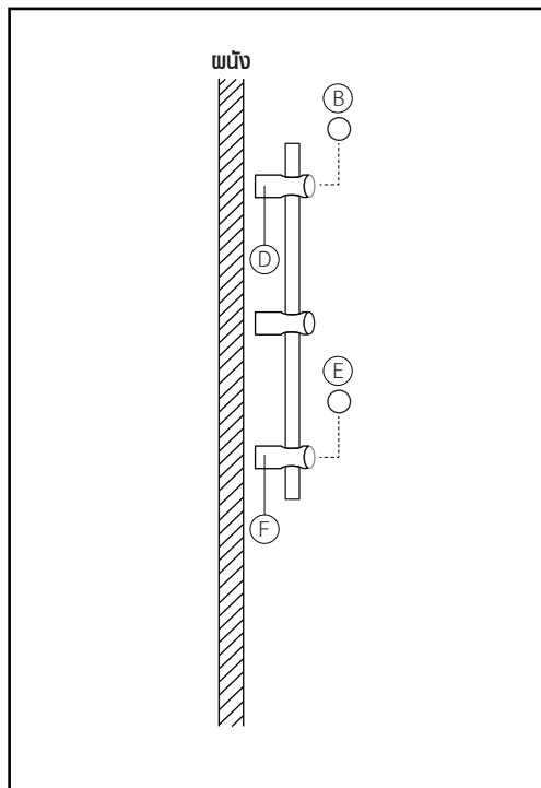
4. ใส่ฝาคกรอบเป็น ( B,E ) เข้ากับแป้นด้านบน ( D ) และด้านล่าง ( F )
