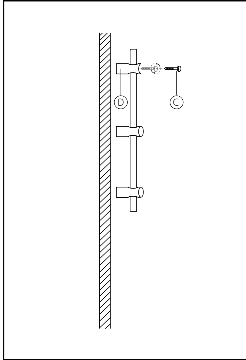
2. เปิดฝาคกรอบเป็นด้านบน ( B ) เพื่อนำสกรู ( C ) ใส่ไปด้านในเป็นบน ( D ) และขันสกรูยึดแป้นเข้าผนัง
