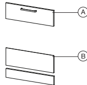
Art. 1281860 บานลีนชักโครงตุลาง W60 x D2 x H18 CM. (หน้าบาน) (A) W60 x D2 x H20 CM. (หน้าบาน) (B) W60 x D2x H10 CM. (แผ่นปิดชาตุ้)
