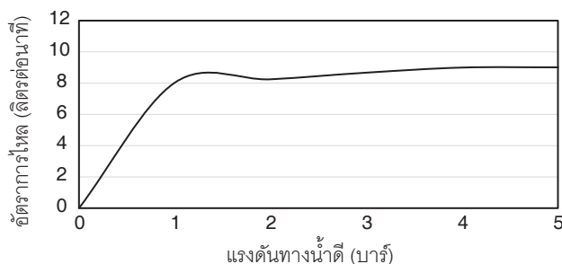
กราฟแสดงอัตราการไหล (K-26294T)
