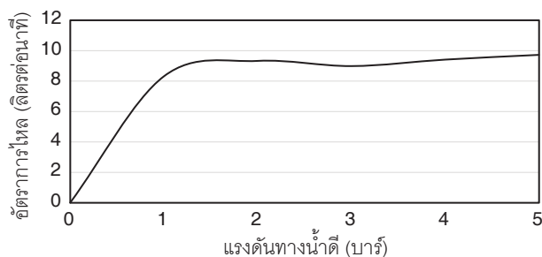
กราฟแสดงอัตราการไหล (K-26292T)
