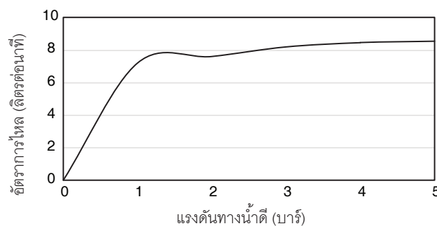
กราฟแสดงอัตราการไหล ฝักบัวสายอ่อน สำหรับ BL
