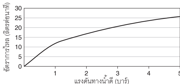
กราฟแสดงอัตราการไหล ฝักำบัวสายอ่อน
