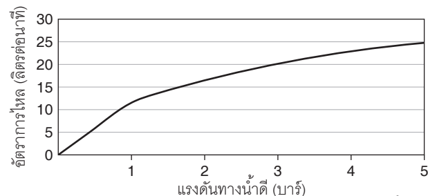
กราฟแสดงอัตราการไหล ก๊อกลงอ่างอาบน้ำ
