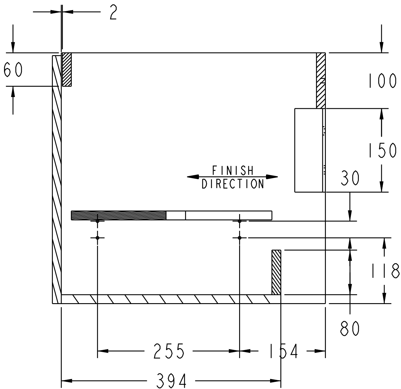
SECTION A-A
