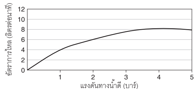
กราฟแสดงอัตราการไหล K-25103T-4CD
