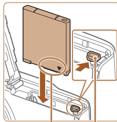
Đầu cực Khóa pin
